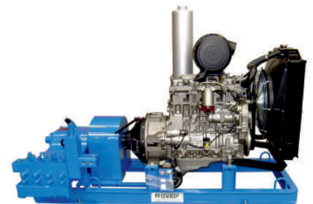
3100A02 - 100 CV 280 bar - 135 l/min
