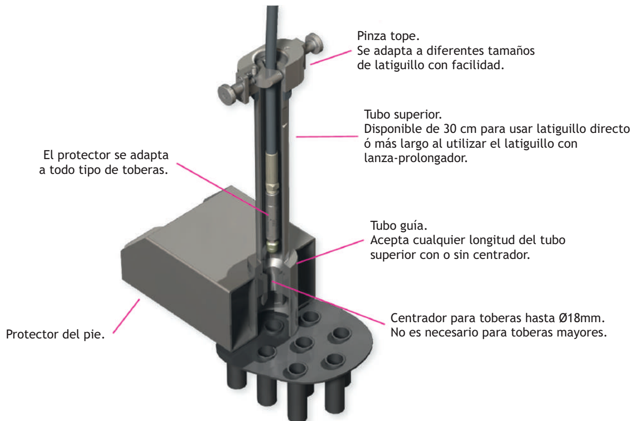
Pinza tope del latiguillo
