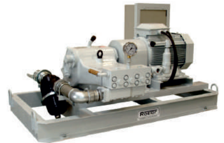
3150RB02 - 50 CV 60 bar - 322 l/min
