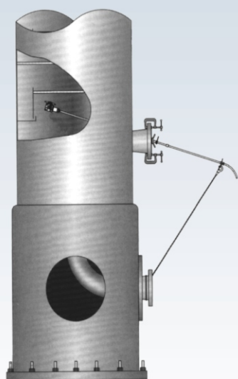
Torre destilación
